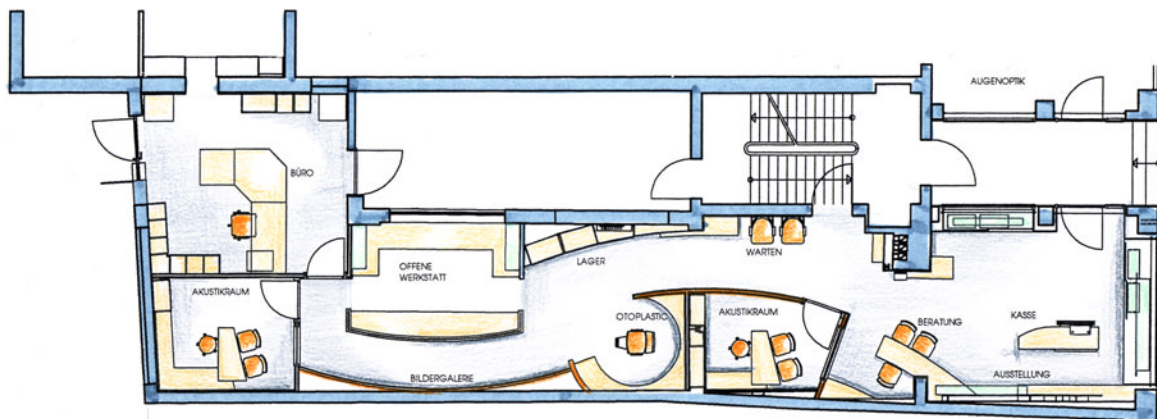
Hilgenfeld Hörakustik ■ Stadthagen Grundriss
